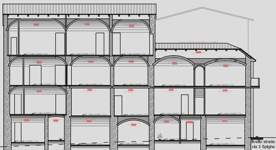
SEZIONE B-B
